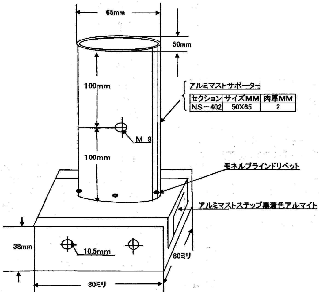
アルミマストステップ船体取り付け寸法図
